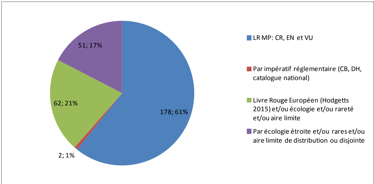
Figure 1. Bryophytes déterminantes pour les ZNIEFF selon les différents cas considérés.
