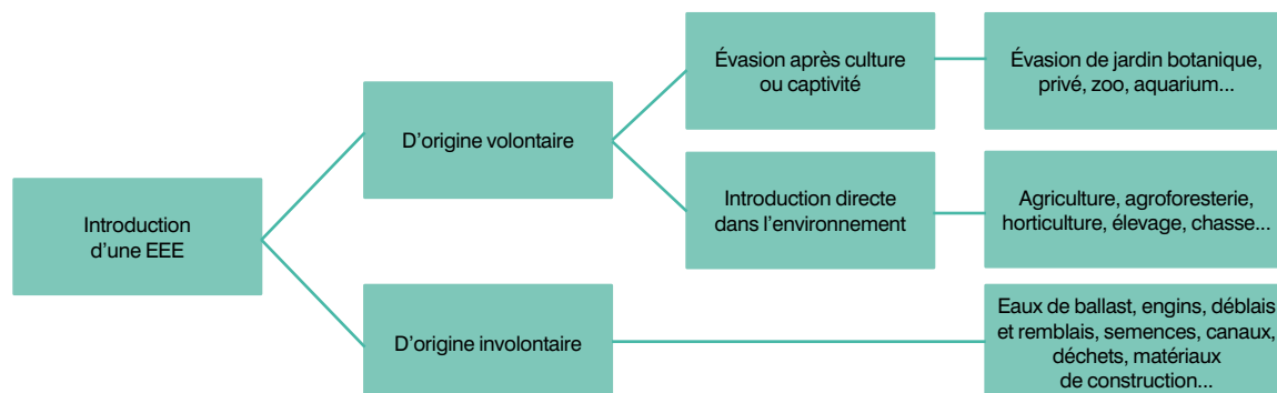
Fig. 1 : Modes d'introduction des espèces exotiques envahissantes. D'après Soubeyran, 2008.
