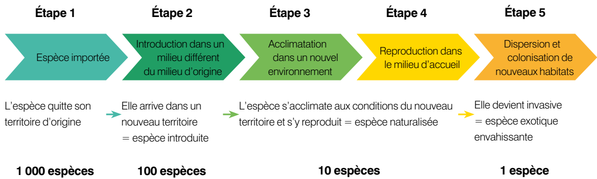
Fig. 2 : Schéma théorique de la dynamique des espèces conduisant à des invasions biologiques. D'après Richardson et al., (2000) et Williamson (1996)
