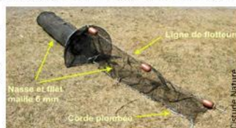
Nasse à simple entrée avec filet
