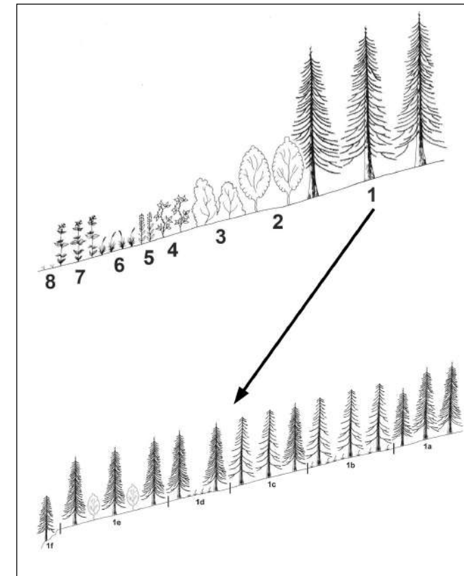
Figure 4. En haut, modèle théorique de la série montagnarde de l'épicéa ( Picea abies ) [ Luzulo nemorosae-Piceetum ] ; 1 – forêt ( Luzulo nemorosae-Piceetum ) ; 2 – bas-manteau ( Salicetum capreae ) ; 3 – bas manteau ( ) ; 4 – broussaille ( Rubetum idaei ) ; 5 – Epilobietum angustifolii ; 6 – pâturage ( Sieversio-Nardetum strictae ) ; 7 – végétation des cultures de pommes de terre ( Galinsogo-Portulacetum ) ; 8 – végétation pionnière ; En bas phases de dégénération de l'association Luzulo nemorosae-Piceetum ; 1a forêt normale en régénération ; 1b – pâturages à mélèze ( Larix decidua ) – mélèzins ; 1c – reboisements anciens de Larix decidua ; 1d – clairières dans la forêt avec prairies du Sieversio-Nardetum strictae ; 1e clairières dans la forêt avec Alnus incana produit de la succession secondaire ; 1f – forêt ouverte à cause d'érosion par gravité.
