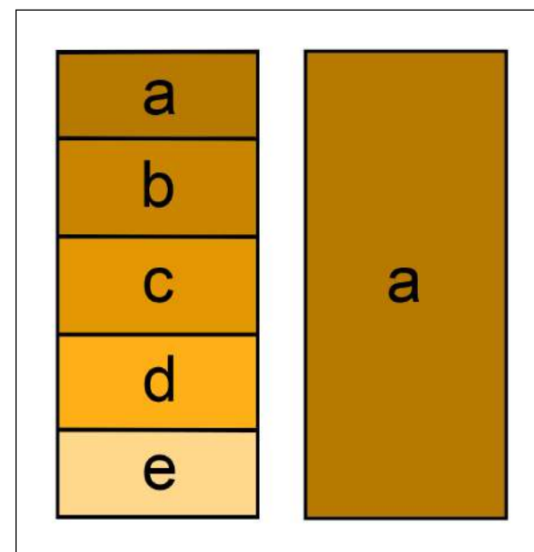
Figure 3. Utilisation des couleurs pour la représentation cartographique de la série ; à gauche, sont représentés tous les stades de la série (représentation analytique), à droite, seule l'association tête de la série (représentation synthétique).
