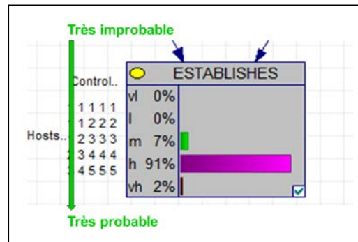
Figure 20 : Evaluation (au moyen de l'application GeNle) de la probabilité d'établissement d' O. communa
