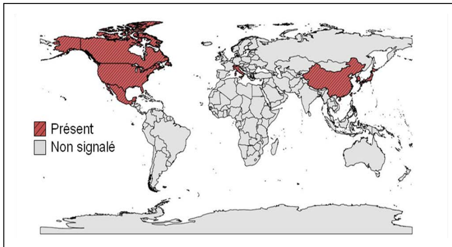
Figure 4 : Distribution d' Ophraella communa au niveau mondial
