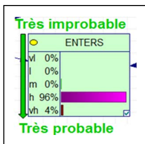
Figure 12 : Evaluation de la probabilité d'entrée par dissémination naturelle d' O. communa
