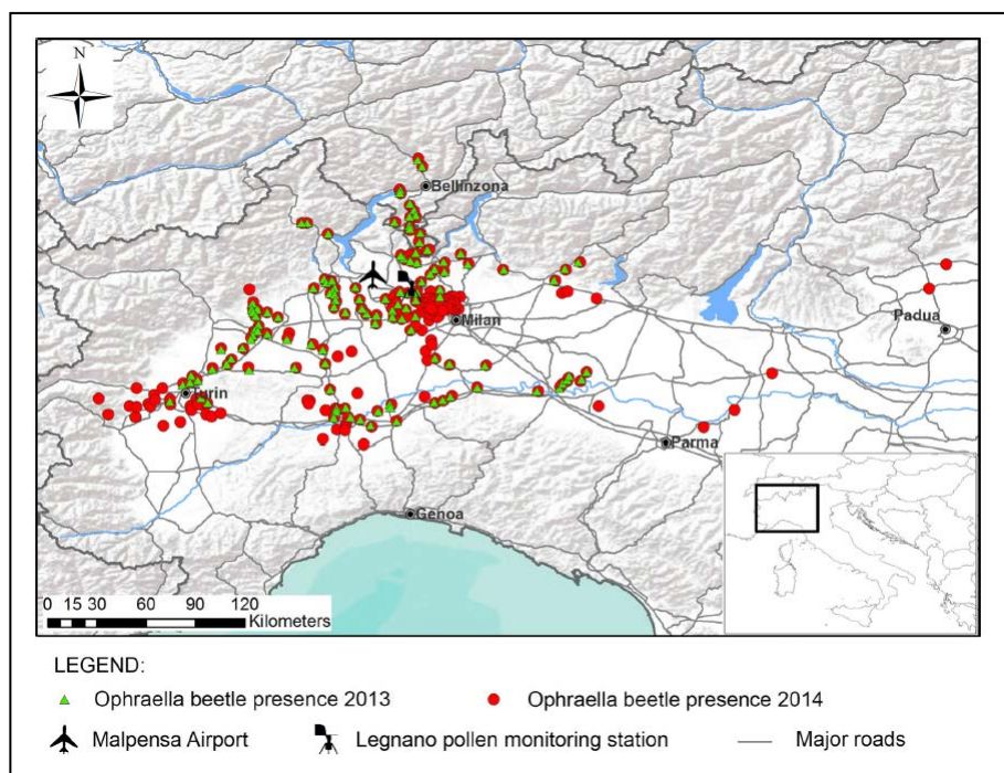
Figure 5 : Distribution d' Ophraella communa en Europe en 2013 et 2014 (Bonini et al. , 2015a)
