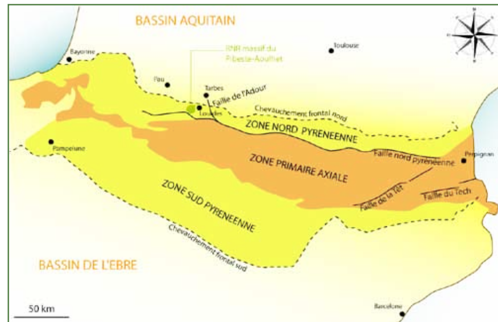
Figure 10 : Carte illustrant la structure géologique des Pyrénées
