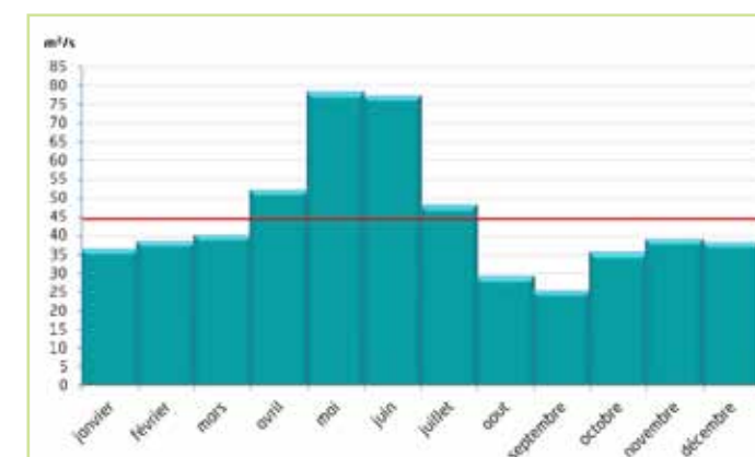
Figure 8 : Débits moyens mensuels mesurés du Gave de Pau à Saint-Pé-de-Bigorre de 1972 à 2012 (surface du bassin versant = 1 120 km 2 ) Source: Banque Hydro
